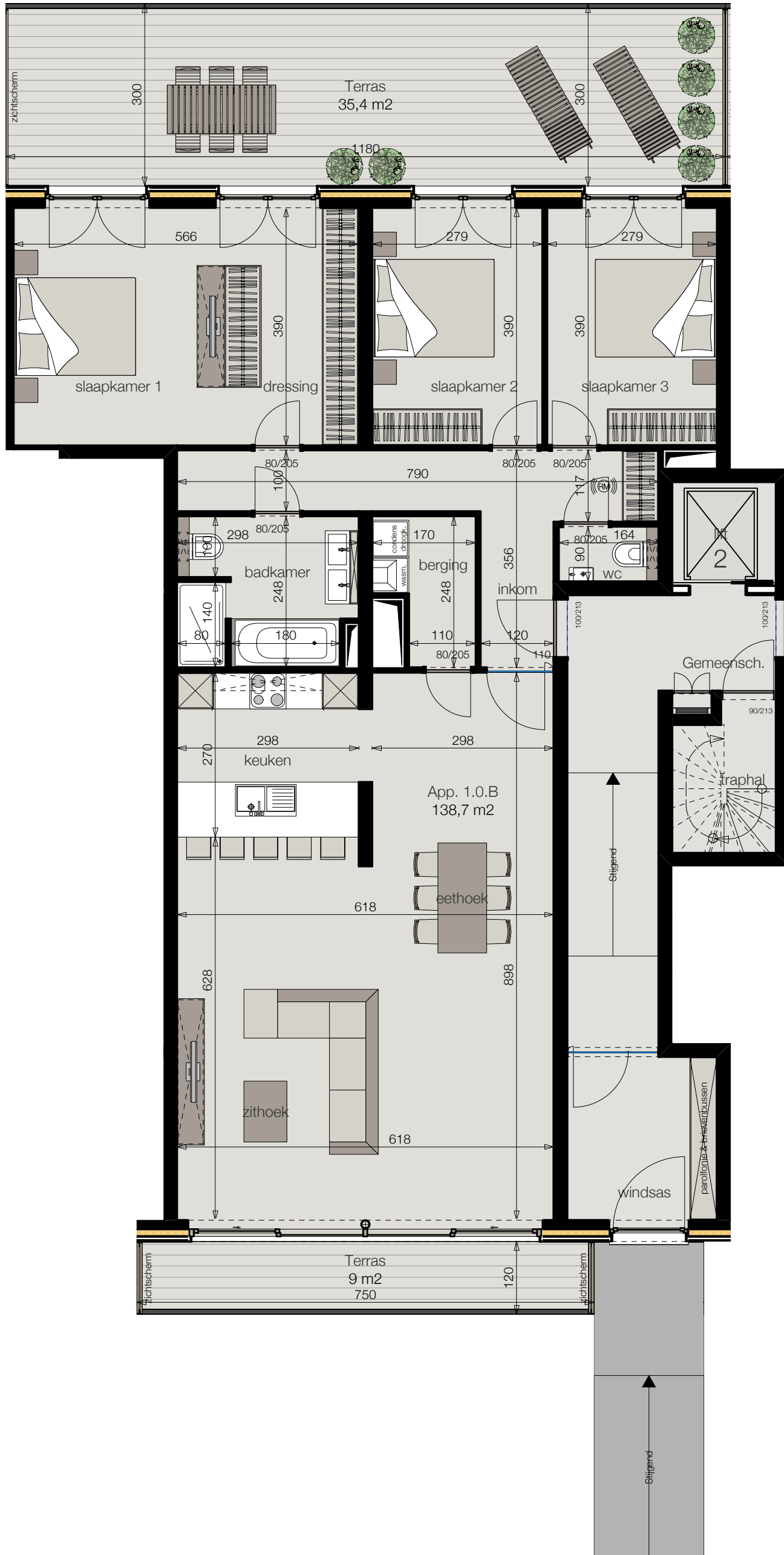
App. 1.0.B Schaal: 1:75
